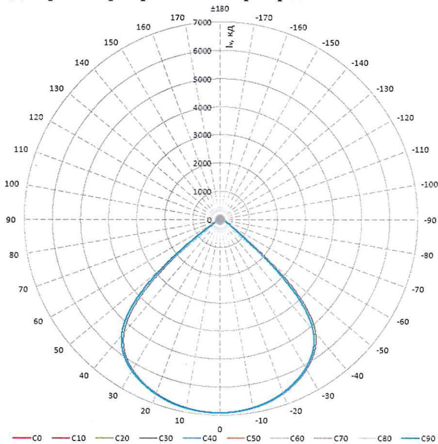
Диаграмма пространственного распределения силы света
